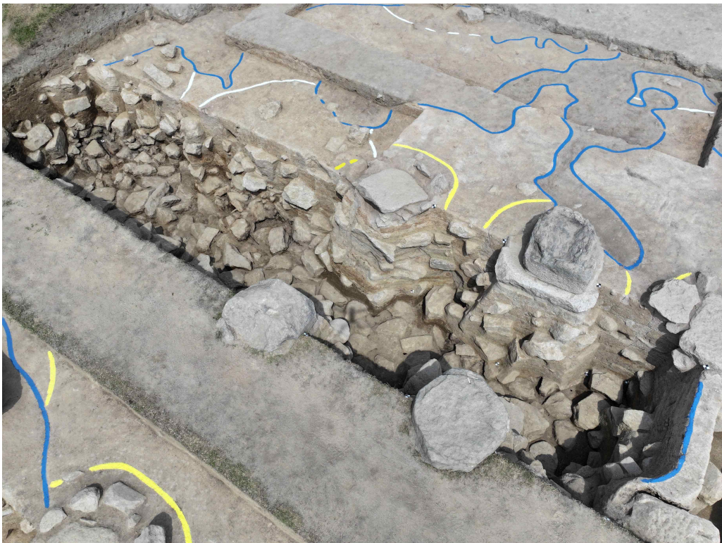
<익산 미륵사 중원 금당지 기둥 기초 구조(서남에서)>
