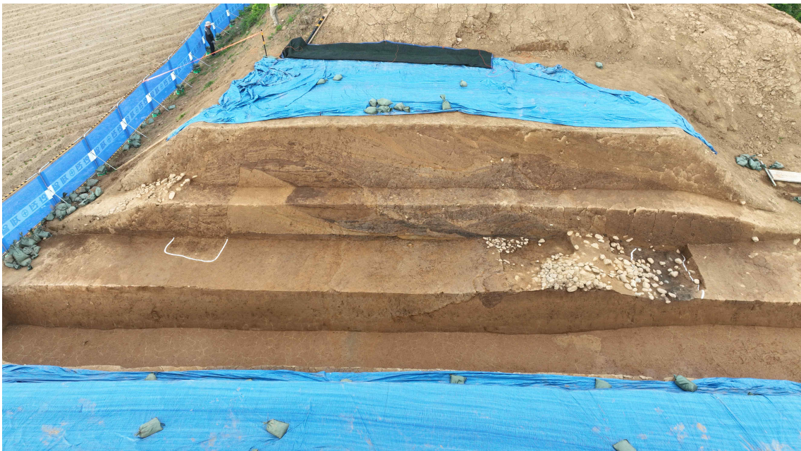
<2024 파주 육계토성 남성벽 조사구간 전경>
